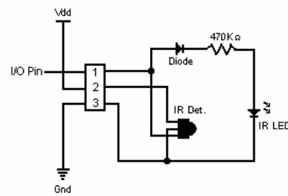
Fig. 13 - IR schematic
