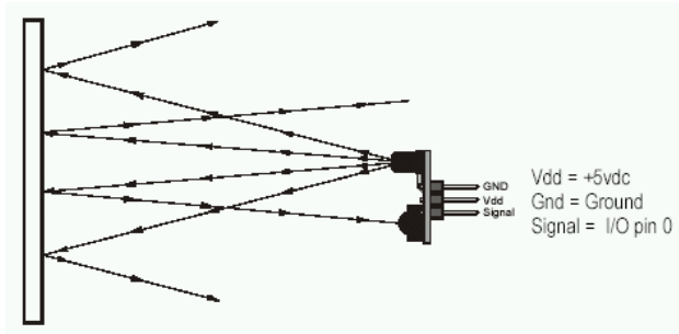
Fig. 12 - IR specification
