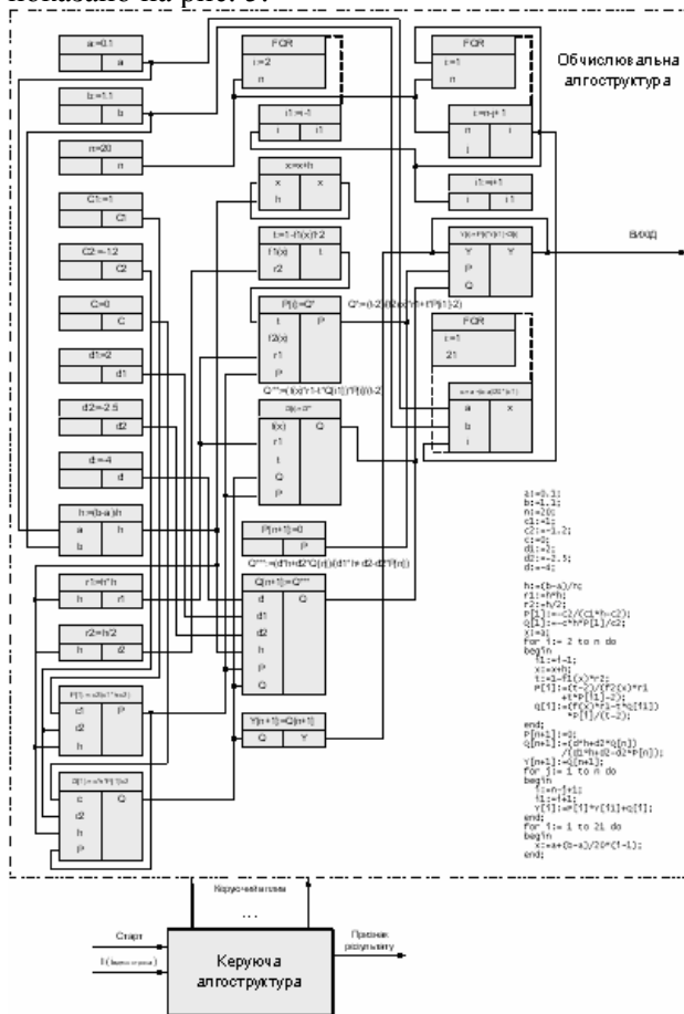
Рис. 3 – Алгоритмична структура для крайової задачі методом прогонки
