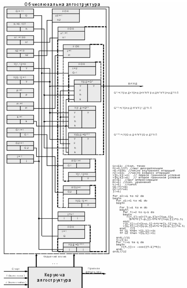
Рис. 4 – Алгоритмична структура для крайової задачі на підставі точкових обчислень
